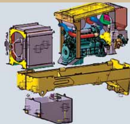
Projeto dos componentes tipo modular
